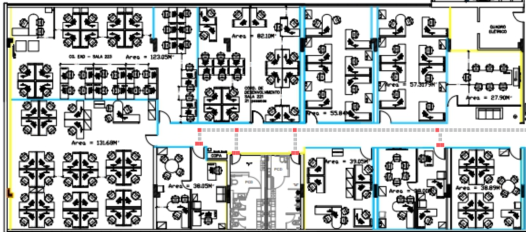
PLANTA BAIXA - BLOCO PRINCIPAL -2º PAVIMENTO
